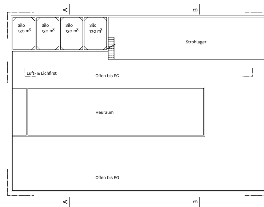
Grundriss Obergeschoss
