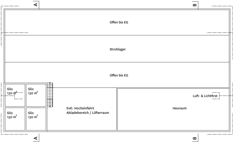
Grundriss Obergeschoss
