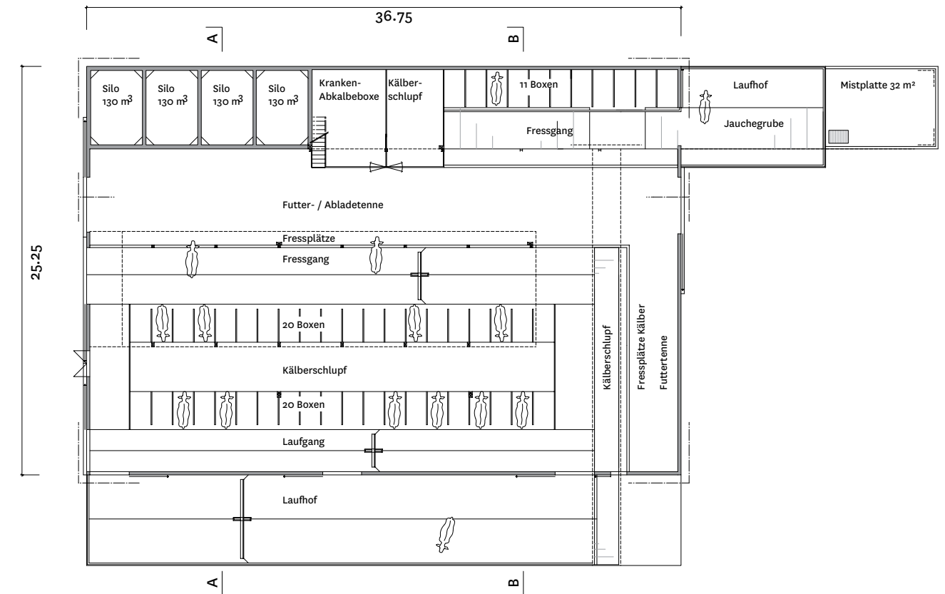
Grundriss Erdgeschoss
